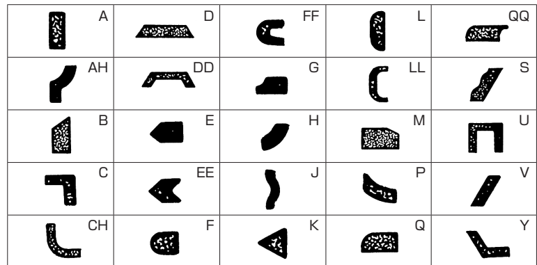
図 3 ダイヤモンド層の断面形状
