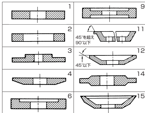
図 2 台金の基本形状
