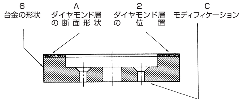
図 3 ダイヤモンド層の断面形状
