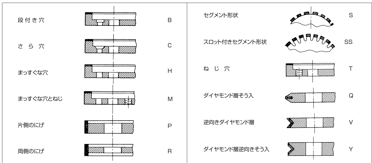
図 5 モディフィケーション
