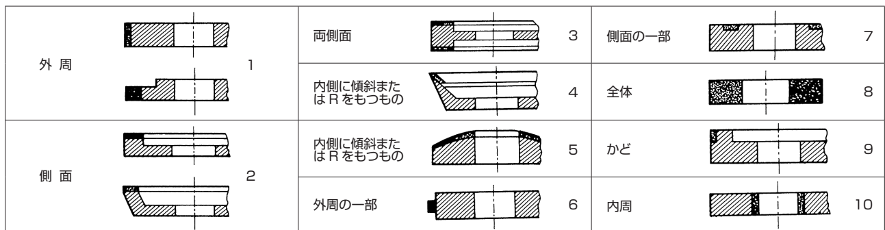
図 4 ダイヤモンド層の位置
